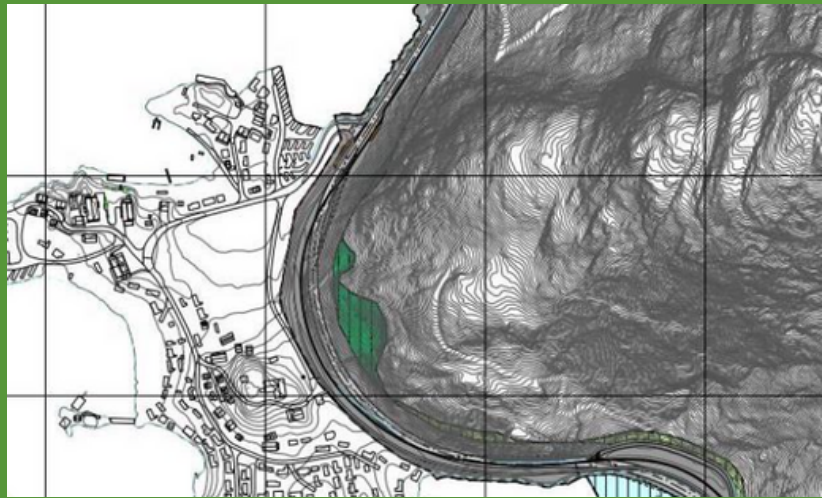
KURVEUTBETRING, RV. 9 NESET CAMPING
